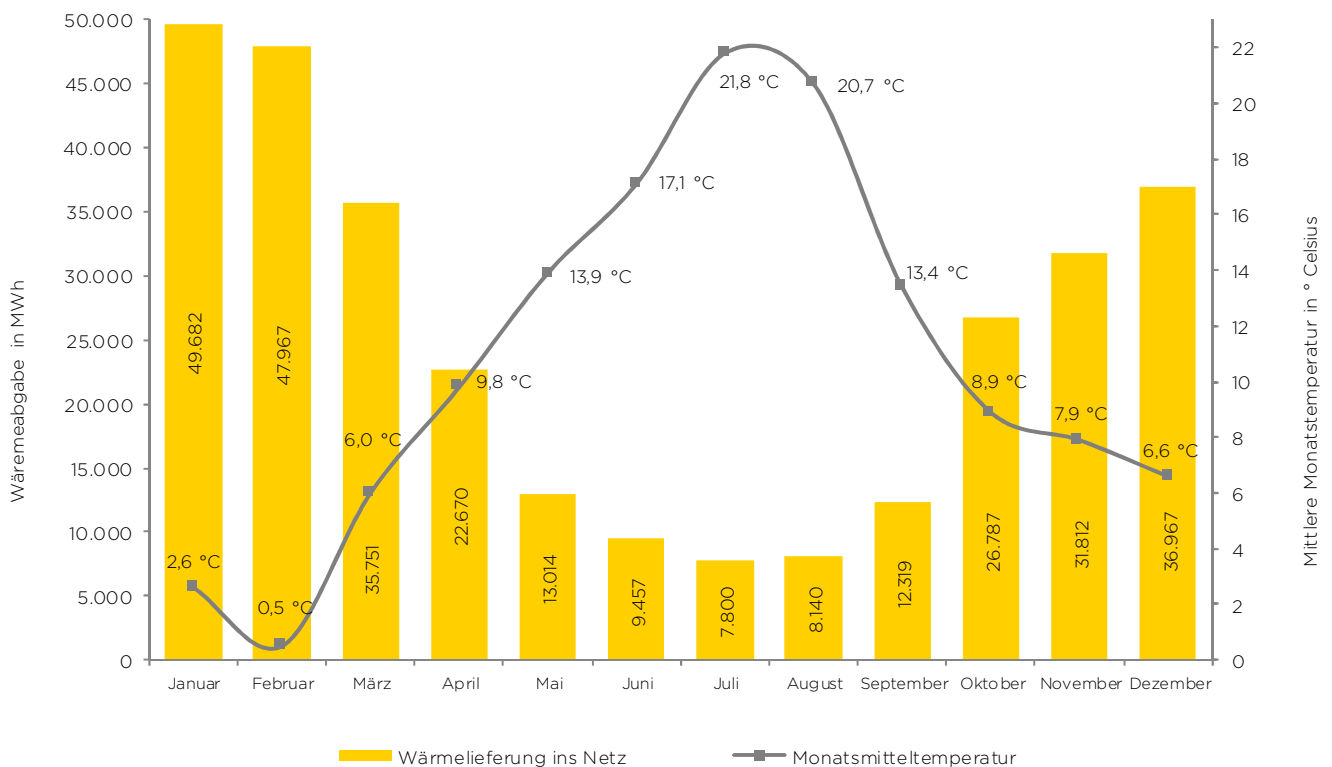
Monatsmitteltemperatur und Wärmeabgaben der Stadtwerke Pforzheim im Jahr 2015
